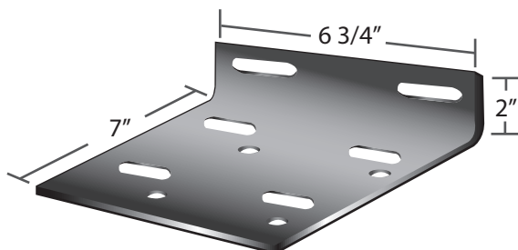
Placa "L" de montaje
